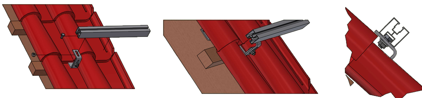
WIDOK DACHU Z ZAMONTOWANYM PROFILEM KBH-PV-01
